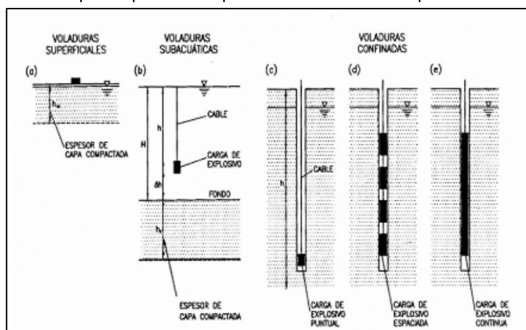
Figura 5 Esquema para la compactación del suelo con explosivos
