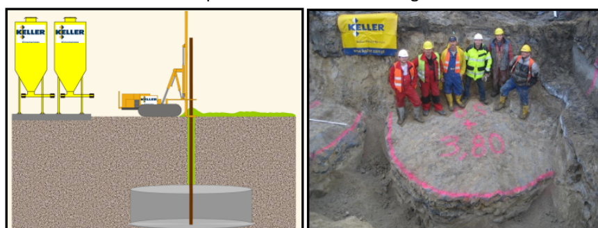
Figura 6 Implementación de Jet Grouting
