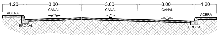
SECCION TRANSVERSAL TIPO ESC: 1:100
