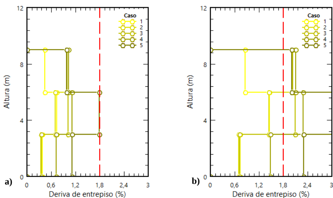
Figura 10. Derivas de entrepiso de edificio de 3 niveles según procedimiento: a) Estándar y b) Alternativo
