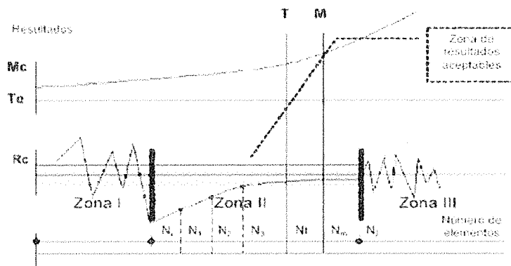
Figura 2- 20. Variación del resultado por variación de número de elementos, tomado de Elberg y Febres. [21]
