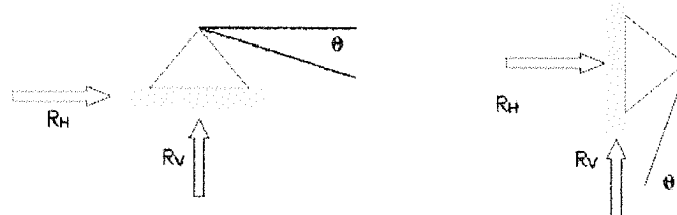
Figura 2- 24. Representación de reacciones y movimientos permitidos en apoyo fijo
