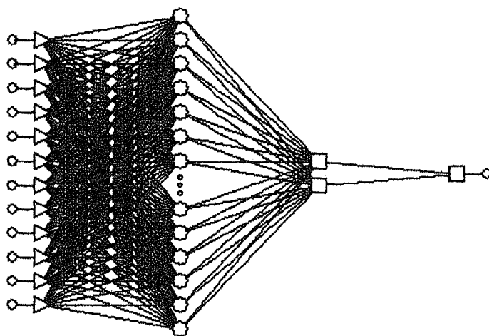
Figura 7- 9. Imagen representativa de la red neuronal artificial donde muestra las doce entradas, energía de deformación, magnitud y fecha con cuatro retardos cada una, y la única salida solicitada.
