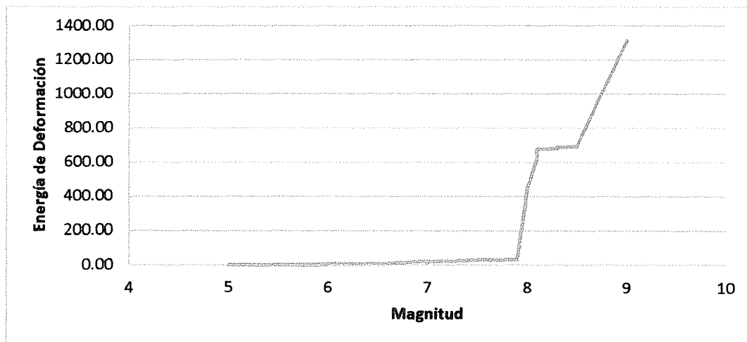
Figura A- 11. Variación de la Magnitud en función la Energía de Deformación en Zona E.
