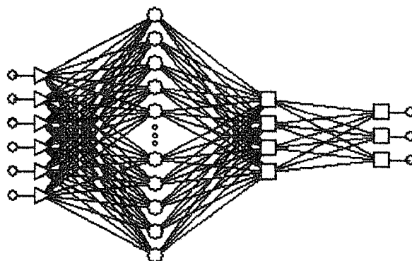
Figura 7- 8. Imagen representativa de la red neuronal artificial donde muestran las seis entradas, energía de deformación, magnitud y fecha con dos retardos cada una, y las tres salidas.
