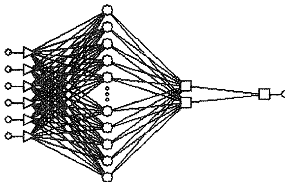
Figura 7- 6. Imagen representativa de la red neuronal artificial donde muestran las seis entradas, energía de deformación, magnitud y fecha con dos retardos cada uno, y una sola salida.
