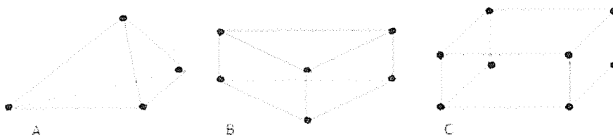
Figura 2- 11. Elementos tridimensionales de cuatro (A), seis (B) y ocho (C) nodos.
