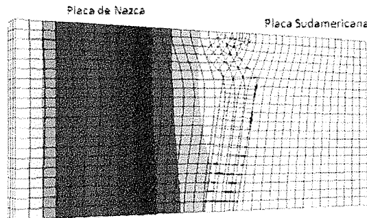
Figura 4- 4. Modelo 2. Muestra las placas Nazca y Sudamericana en 3D, choque frontal.
