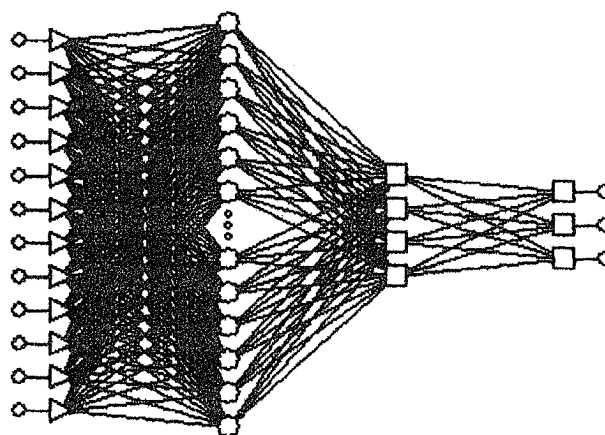
Figura 7- 11. Imagen representativa de la red neuronal artificial donde muestra las doce entradas, energía de deformación, magnitud y fecha con cuatro retardos cada una, y las tres salidas solicitadas.
