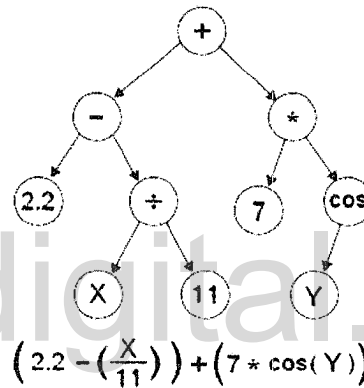
Figura 2- 51. Un individuo en la PG, que representa la expresión matemática indicada en la parte inferior de la figura
