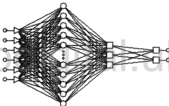
Figura 7- 7. Imagen representativa de la red neuronal artificial donde muestran las seis entradas, energía de deformación, magnitud y fecha con dos retardos cada una, y dos salidas.
