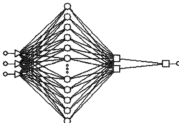
Figura 7- 2. Imagen representativa de la red neuronal artificial donde muestra tres entradas: energía de deformación, magnitud y fecha, y una sola salida.
