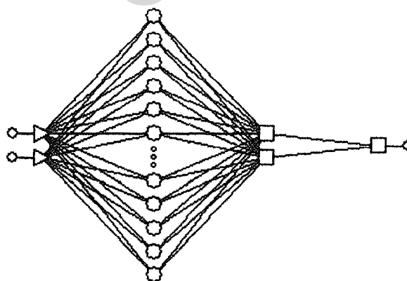
Figura 7- 1. Imagen representativa de la red neuronal artificial donde muestra dos entradas: magnitud y fecha, y una sola salida.
