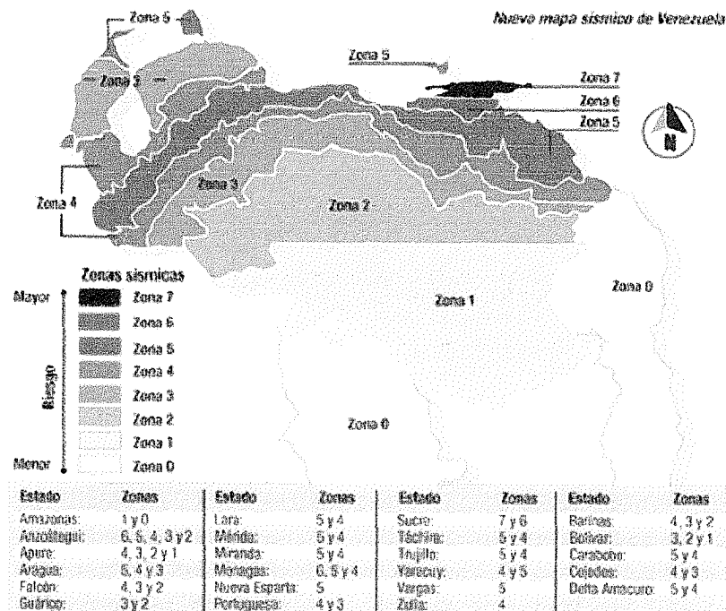
Figura 8- 24. Zonas sísmicas de Venezuela de las normas para la construcción de edificaciones civiles.
