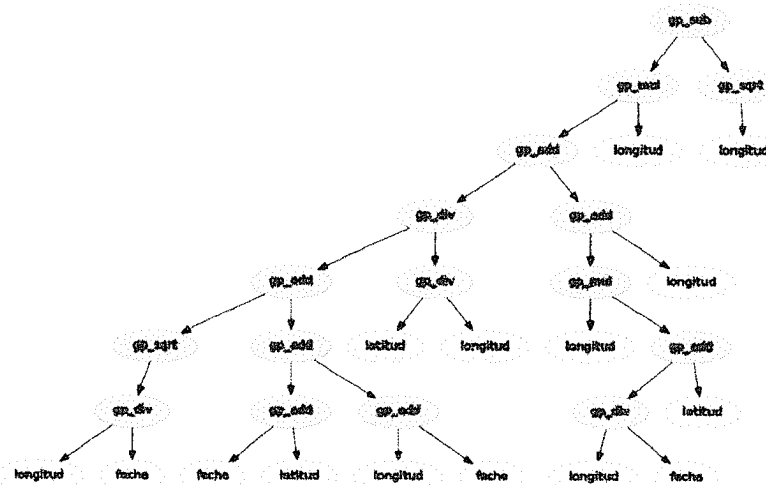
Figura 6- 4. Árbol de la Falla de Boconó
