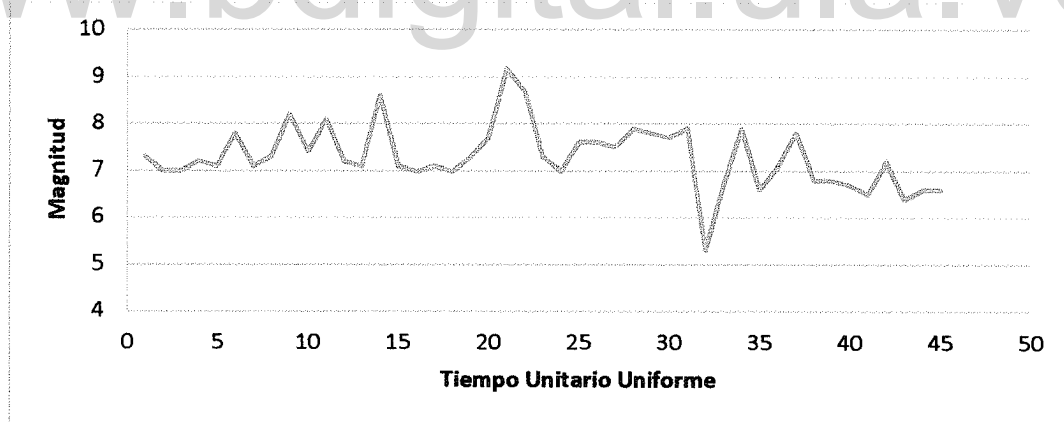
Figura A- 8. Variación de la Magnitud en función del Tiempo Unitario Uniforme en Zona F.
