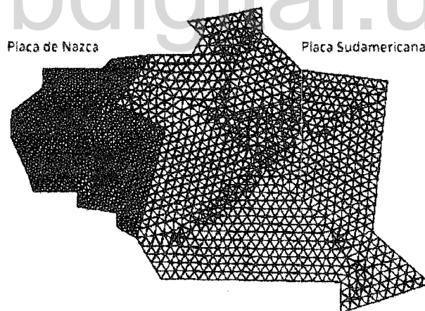
Figura 4- 3. Modelo 1. Se muestra la placa de Nazca y la placa Sudamericana.
