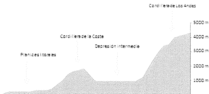
Figura 8-19. Relieve de Zona Central de Chile, 33° de latitud Sur
