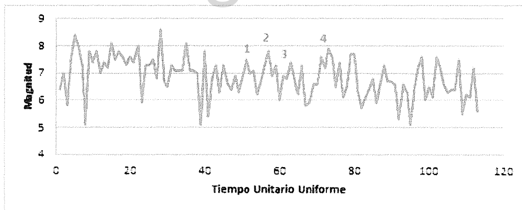
Figura A- 2. Variación de la Magnitud en función del Tiempo Unitario Uniforme en Zona C.
