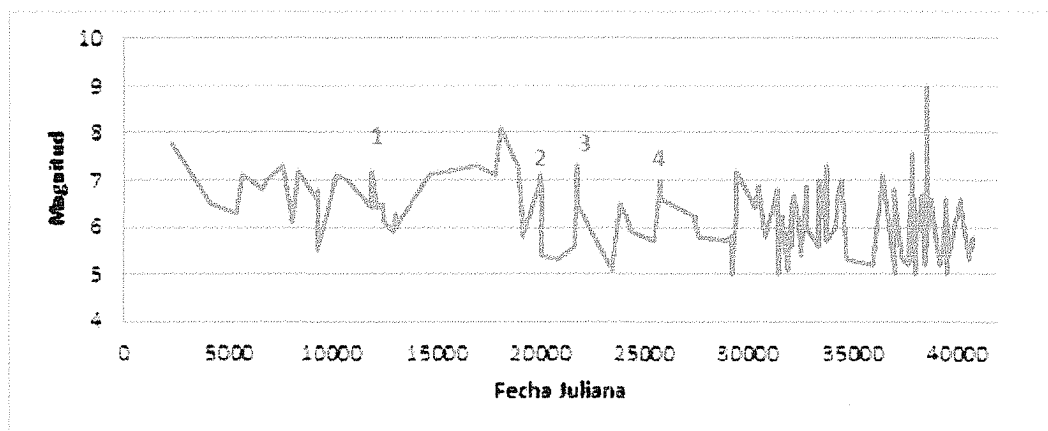
Figura A- 3. Variación de la Magnitud en función de la Fecha Juliana en Zona D.
