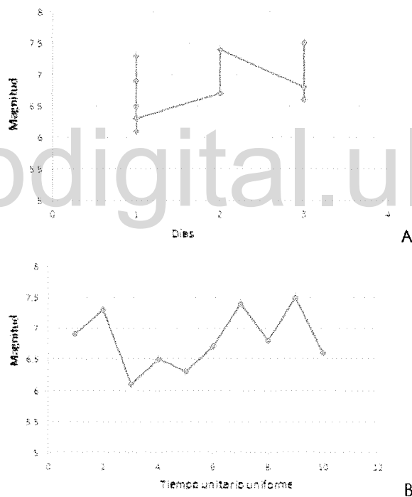
Figura 8-1 A y B. Representación de datos sísmicos, en la primera figura se muestran los tres días de datos. En la segunda figura se muestran los 10 datos.
