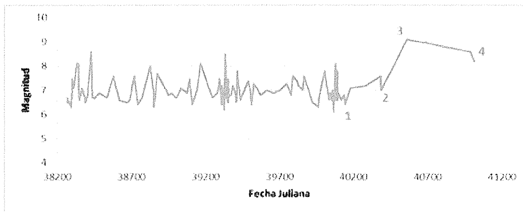
Figura 8- 4. Variación de la Magnitud en función de la Fecha Juliana en Zona B.
