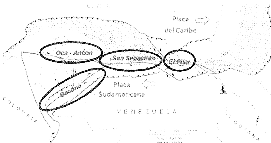
Figura 6- 1. Ubicación de la Falla de Boconó, Falla de San Sebastián, Falla Oca Ancón y Falla El Pilar, en Venezuela
