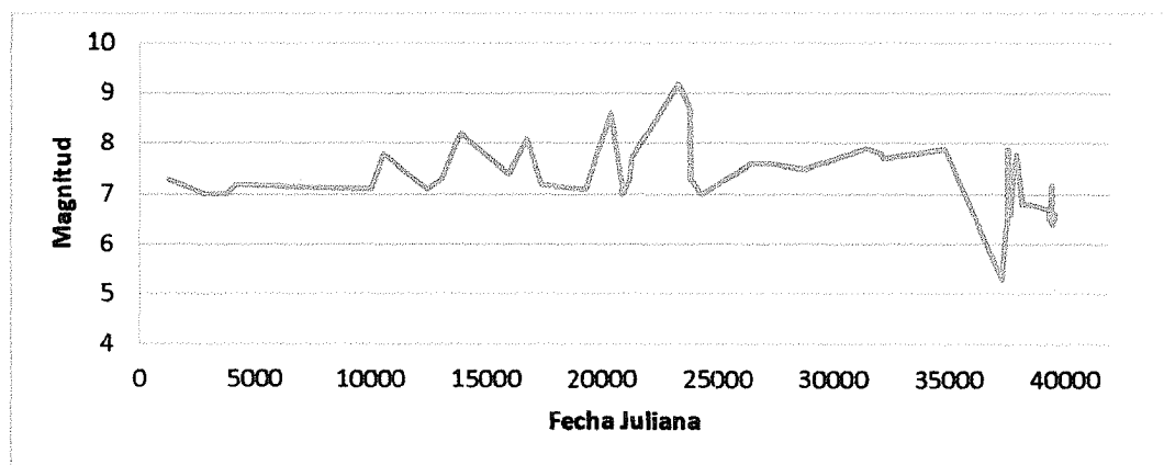
Figura A- 7. Variación de la Magnitud en función de la Fecha Juliana en Zona F.
