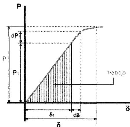
Figura 2- 5. Diagrama carga P – desplazamiento \delta . El área de la franja sombreada debajo de la curva representa el trabajo realizado por la carga. El trabajo total hecho por la carga al pasar de cero al valor máximo P es la suma de todas las franjas elementales, [29].
