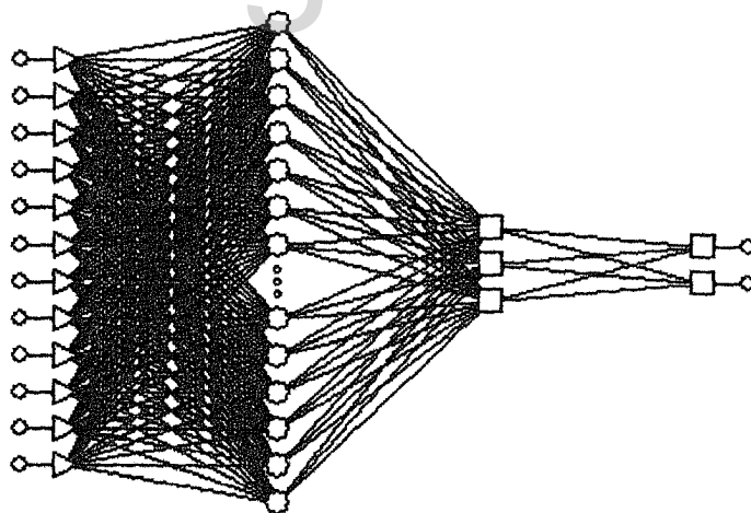
Figura 7- 10. Imagen representativa de la red neuronal artificial donde muestra las doce entradas, energía de deformación, magnitud y fecha con cuatro retardos cada una, y las dos salidas solicitadas.
