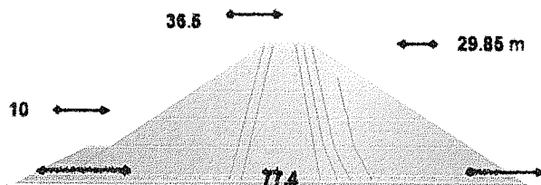
Figura 2- 15. Fotografía de Presa Caruachi y su geometría [14].
