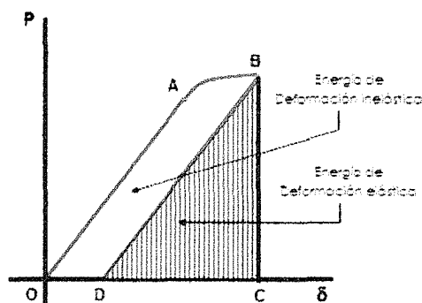
Figura 2- 6. Energía elástica y energía inelástica en el diagrama carga P – desplazamiento \delta . El punto A representa la carga con que el esfuerzo en el material alcanza el límite elástico. [29]
