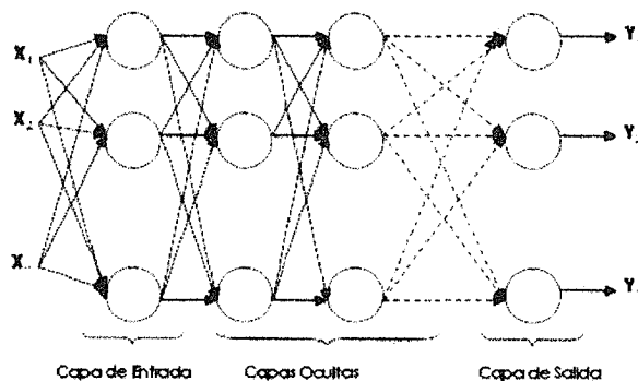
Figura 2- 46. Red perceptrónica multicapa
