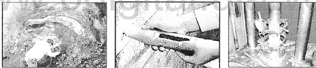
Figura 2- 18. Toma de muestras, medición con esclerómetro in situ y ensayo de compresión uniaxial.
