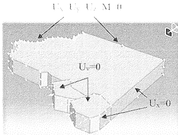
Figura 4- 7. Condiciones de borde utilizadas en la zona C [31]
