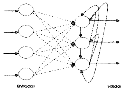
Figura 2- 44 Red con alimentación lateral
