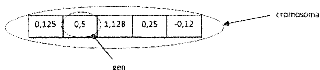
Figura 2- 50. Representación de genes reales
