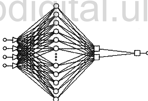
Figura 7- 5. Imagen representativa de la red neuronal artificial donde muestran las cuatro entradas, magnitud y fecha con dos retardos cada una, y una sola salida.
