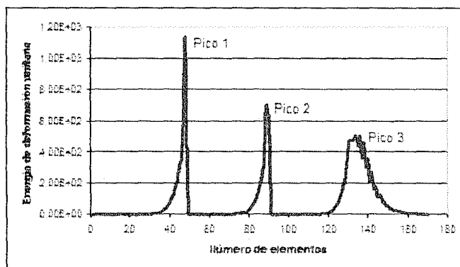
Figura 8-15. Energía de deformación unitaria para 180 elementos seleccionados del modelo por elementos finitos mostrados en el eje X, de la placa Sudamericana del modelo 1
