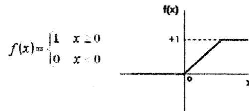
Figura 2- 37. Representación gráfica y grafica de la Función Escalón
