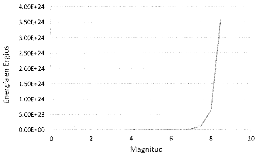
Figura 8-6. Gráfica que representa la variación de la energía en función de la magnitud, utilizando la ecuación 9, [37]
