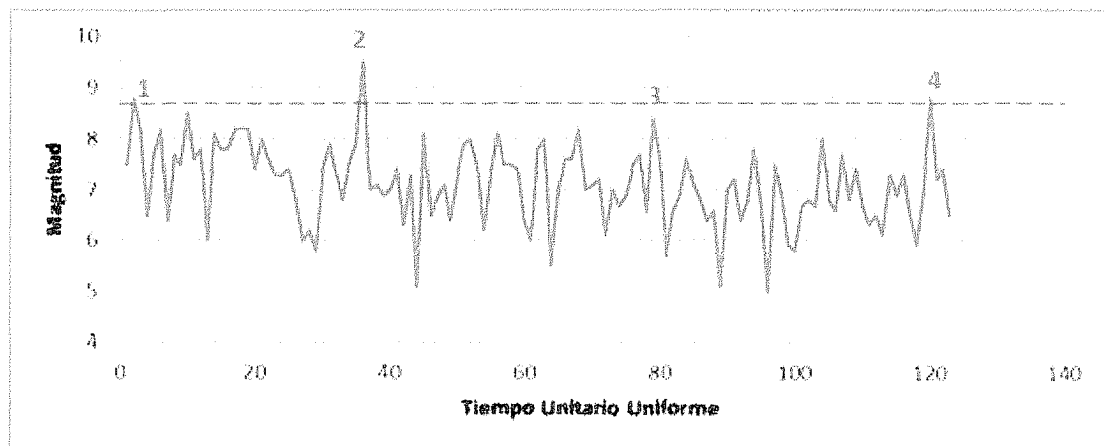
Figura 8-3. Variación de la Magnitud en función del Tiempo Unitario Uniforme en Zona A.
