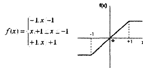
Figura 2- 36. Representación matemática y gráfica de la Función Lineal por tramos
