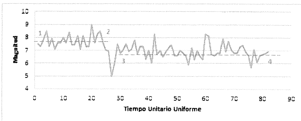
Figura A- 6. Variación de la Magnitud en función del Tiempo Unitario Uniforme en Zona E.
