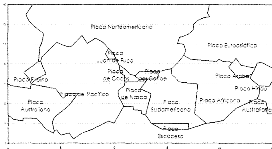
Figura 4- 2. Representación en coordenadas locales de las placas principales de nuestro planeta.
