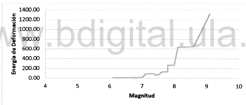
Figura 8-10. Variación de la Magnitud en función la Energía de Deformación en Zona B.
