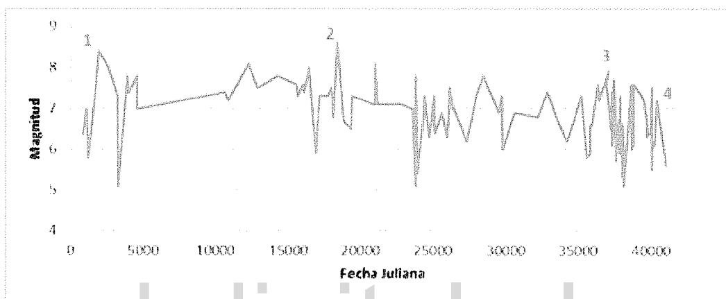
Figura A- 1. Variación de la Magnitud en función de la Fecha Juliana en Zona C.
