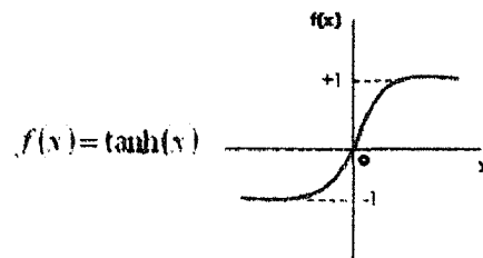
Figura 2- 40. Función Tangencial Hiperbólica
