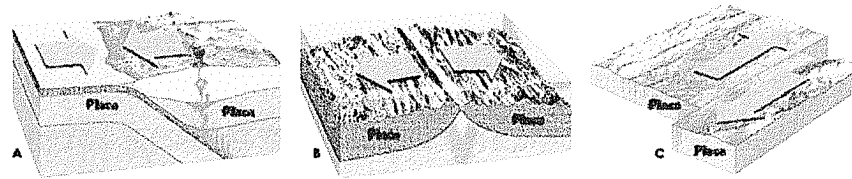
Figura 2- 2. A- Contacto entre placas convergentes, producto de efectos compresivos. B- Contacto entre placas divergentes generados por esfuerzos de tracción. C- Contacto de placas transcurrentes donde no se pierde o gana material. [55]
