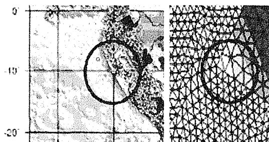
Figura 8-13. Densidad de sismos y distribución de la energía de deformación en zona media, según la simulación geomecánica
