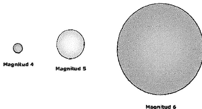
Figura 8-7. Ilustración comparativa que representa la cantidad de energía de un terremoto, por el volumen de una esfera.
