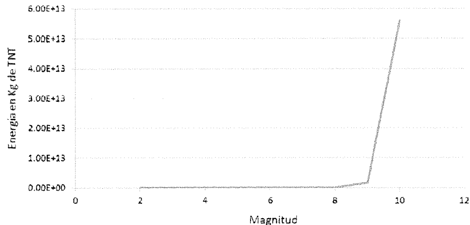
Figura 8-8, Figura que compara la magnitud de los sismos con su equivalente de energía liberada por un poderoso explosivo, TNT, [36].
