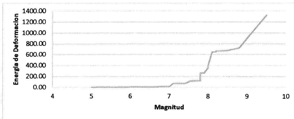
Figura 8-9. Variación de la Magnitud en función la Energía de Deformación en Zona A.
