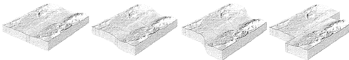
Figura 2- 7. Secuencia de deformación elástica de las rocas, hasta superar los límites de resistencia. [55]
