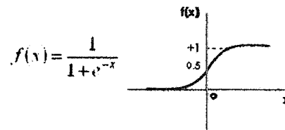
Figura 2- 38. Función Logística o Sigmoidal
