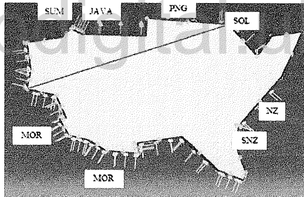
Figura 4- 6. Cargas aplicadas a las Placas Australiana y Filipina. [56]
