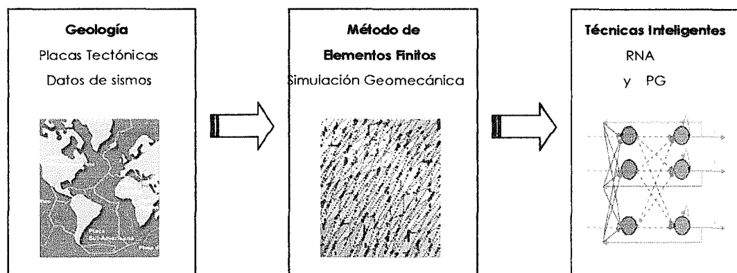
Figura 3- 1. Elementos de la investigación: Geología, Método de Elementos Finitos y Técnicas Inteligentes
