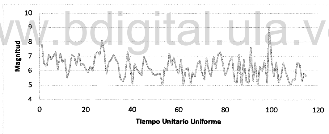
Figura A- 4. Variación de la Magnitud en función del Tiempo Unitario Uniforme en Zona D.
