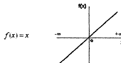
Figura 2- 35. Representación matemática y gráfica de la Función Identidad.
