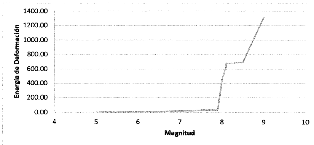
Figura A- 11. Variación de la Magnitud en función la Energía de Deformación en Zona E.
