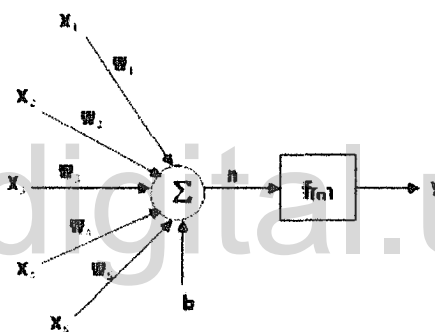
Figura 2- 32. Representación de una Neurona artificial.
