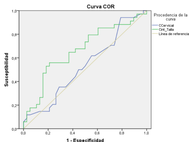
Figura 3. Curva COR para la determinación del punto de corte de la circunferencia de cuello y del índice cintura/talla para predecir el espesor del TAE
