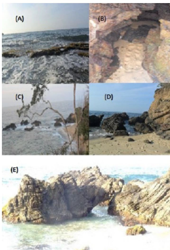
Gráfico 9. Geoformas de erosión en Playa Caimanes. Obsérvese en los detalles: (A) plataforma de abrasión, (B) Cueva submarina, (C) Vista de planta de los farallones, evidenciando hasta donde llegaba el acantilado, (D) Vista de perfil de los farallones, y (E) Arco marino. Nótese en el promontorio ubicado en el extremo inferior derecho de la imagen, los planos de esquistosidad.
