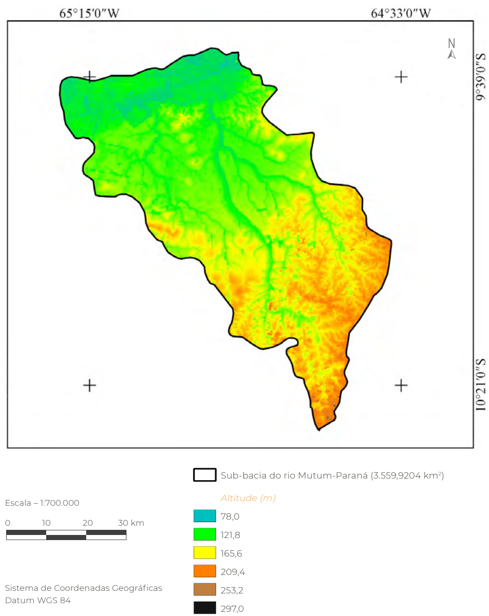
Figura 3 Mapa hipsométrico da sub-bacia do rio Mutum-Paraná, Amazônia Ocidental
