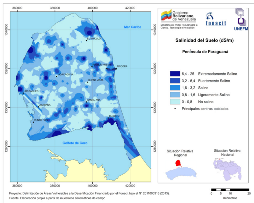
Figura 2. Salinidad del suelo en la Península de Paraguaná.
