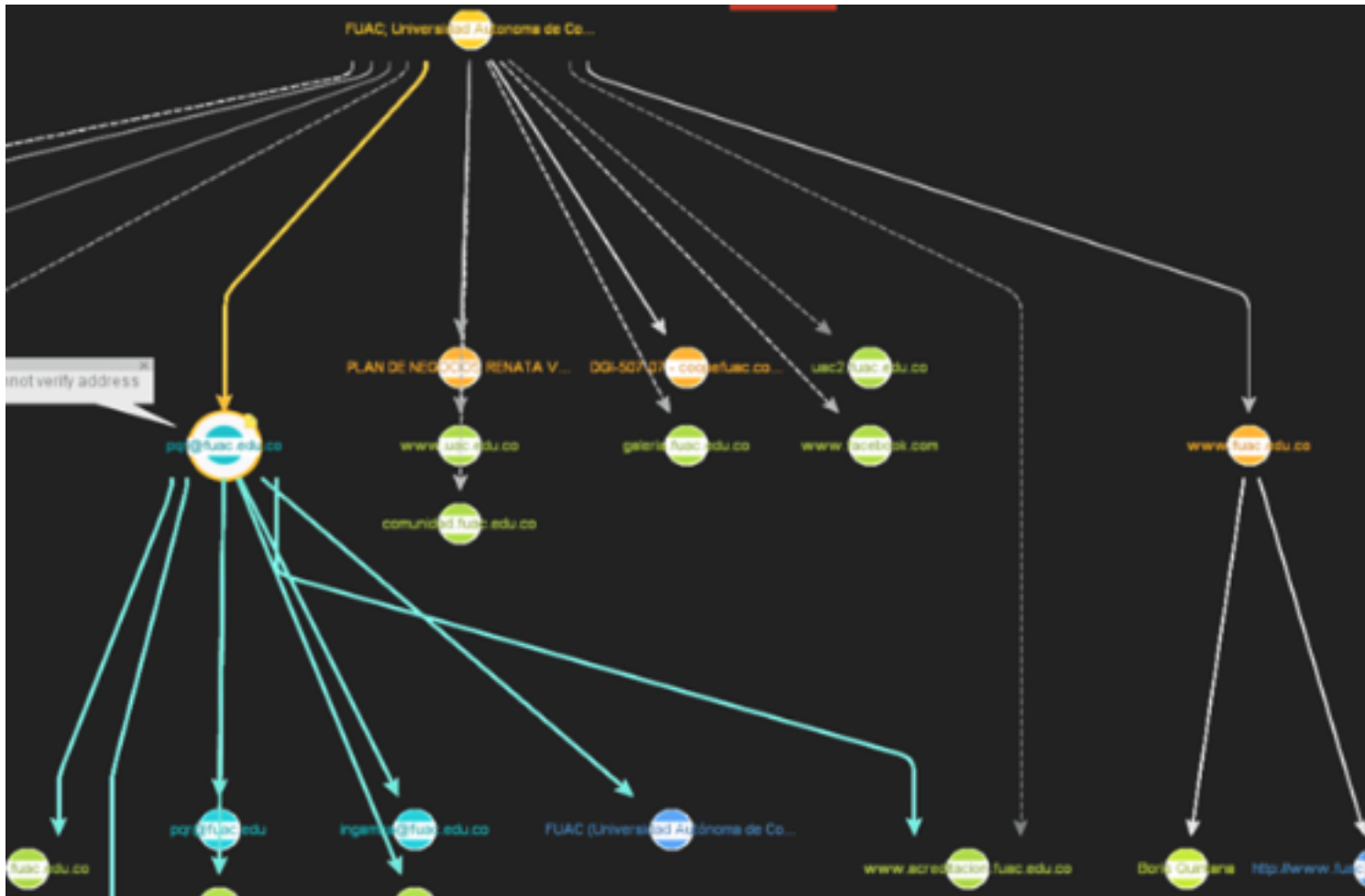
Fig. 3 Grafo generado con Maltego para una dirección de correo electrónico
